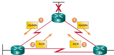
Figur: EIGRP Updatering och bekräftelse[2014snc]
