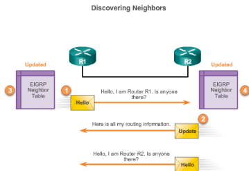
Figur: Upptäcka grannar[2014snc]
