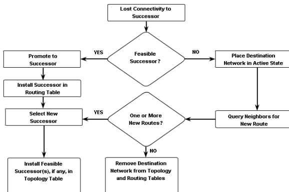
Figur: Flödesdiagram över DUAL FSM[2014snc]
